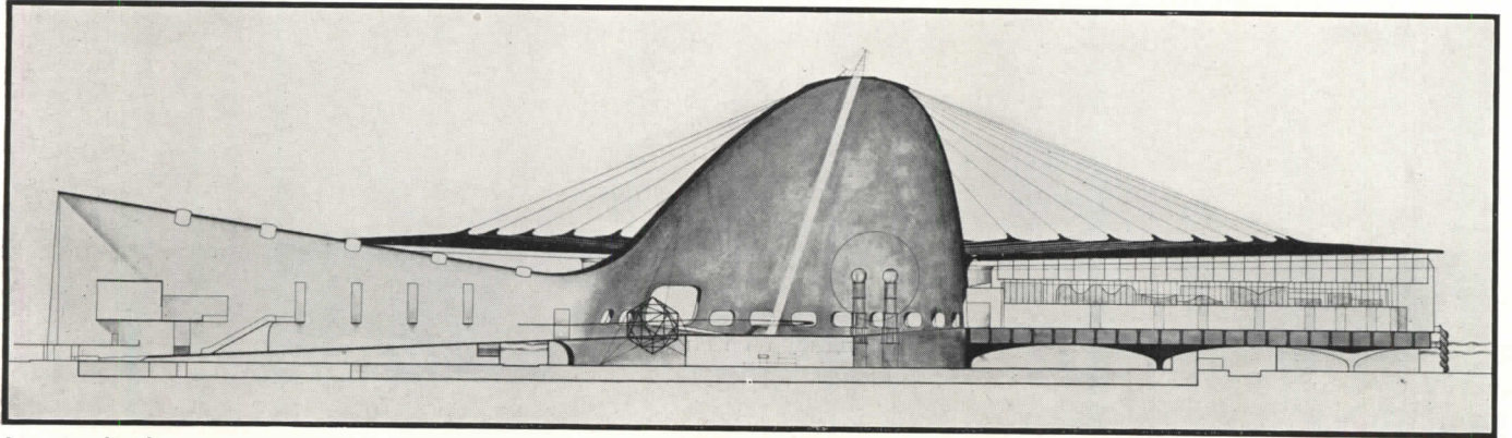
Longitudinal section
