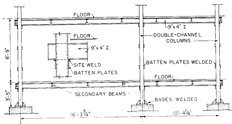
Longitudinal section
